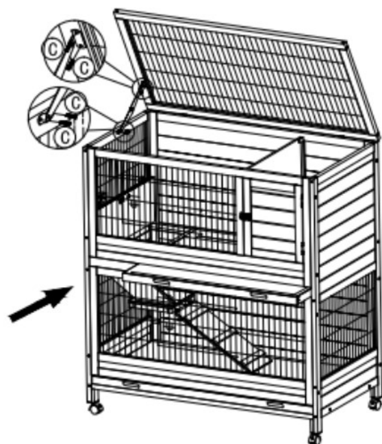
7. insérer le tiroir de déjection haut et fixer la bécuille de toit.
