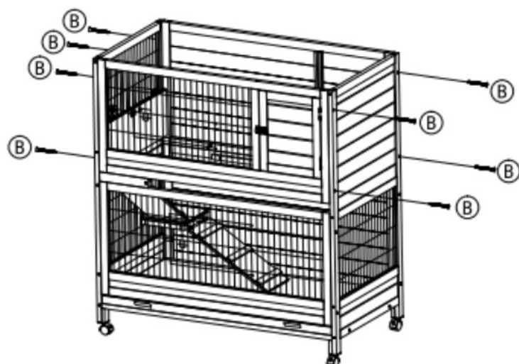
4. fixer le panneau avant haut et la panneau arrière haut.
