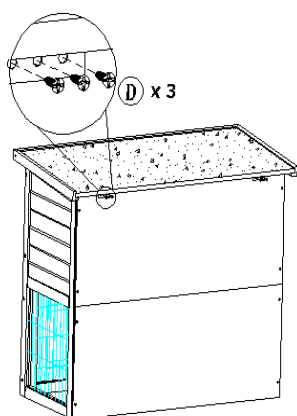
7. Fixer le toit avec les charnières.
