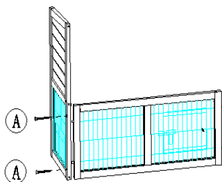
1. Fixer le panneau gauche avec les 2 panneaux avant.
