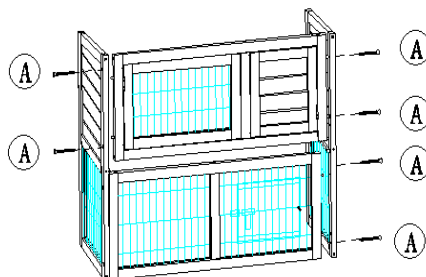
2. Fixer le panneau droit
