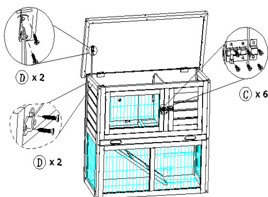
8. Fixer les loquets de fermeture.
