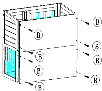
3. Fixer les 2 panneaux arrière.
