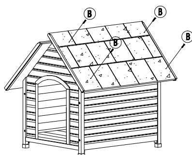
3. Assembler les 2 parties du toit.
